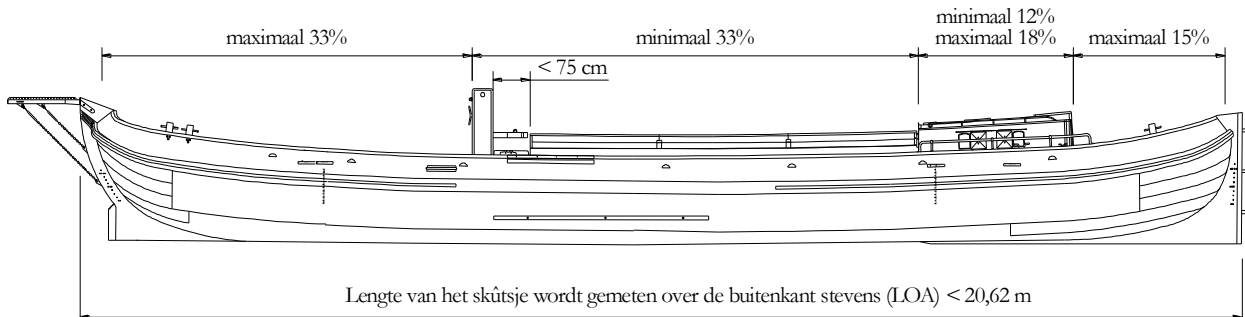
Fig. 2 - Maatvoering skûtsje
