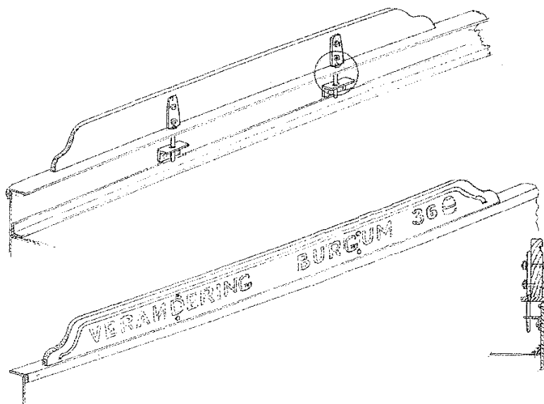
Fig. 8 - Origineel model naambord
