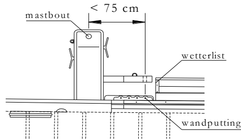
Fig. 10 - Wandputting zijverstaging
